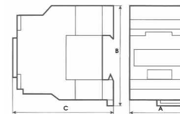
КМЭ -0910; КМЭ -1210; КМЭ -1810
