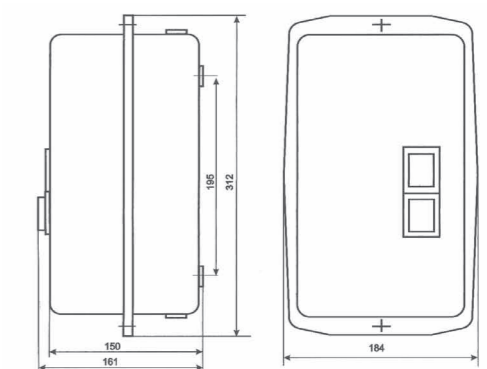
КМЭ(р) 4011; КМЭ(р) 5011; КМЭ(р) 6511; КМЭ(р) 8011; КМЭ(р) 9511
