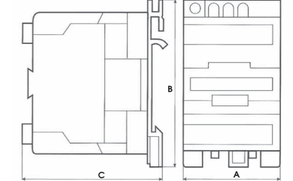
КМЭ -4011; КМЭ -5011; КМЭ -6511
