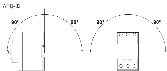
Рабочее положение в пространстве
